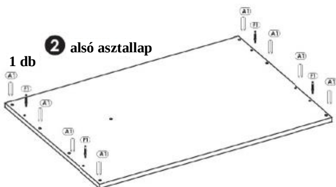
2 alsó asztallap (másik oldal) 1 db
